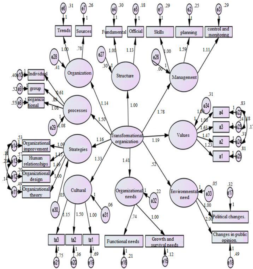
شکل ۳- مدل معادلات ساختاری در حالت غیر استاندارد
