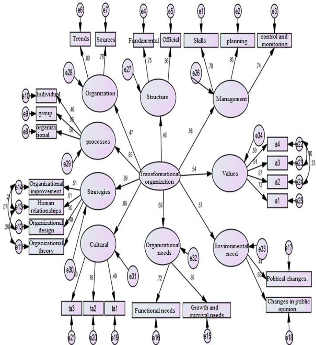
شکل ۲- مدل معادلات ساختاری در حالت استاندارد Figure 2- Structural equation model in standard mode
